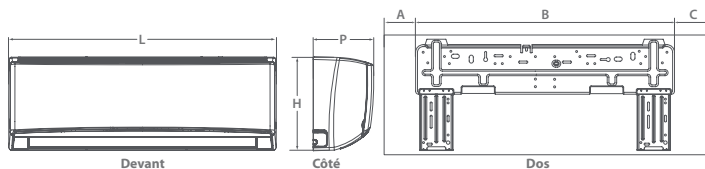
Unité intérieure
